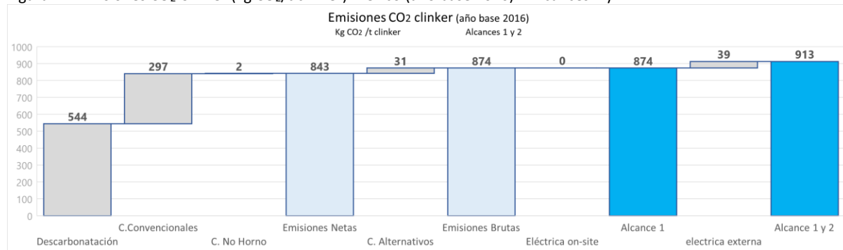
Figura 22. Emisiones CO 2 Clínter (kg CO 2 /t clínter) México (año base 2016) – Alcances 1 y 2
