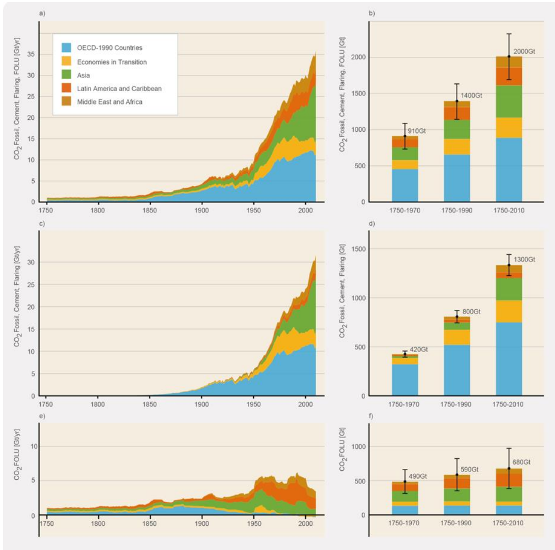
Figura 8. Emisiones antropogénicas históricas de CO 2
