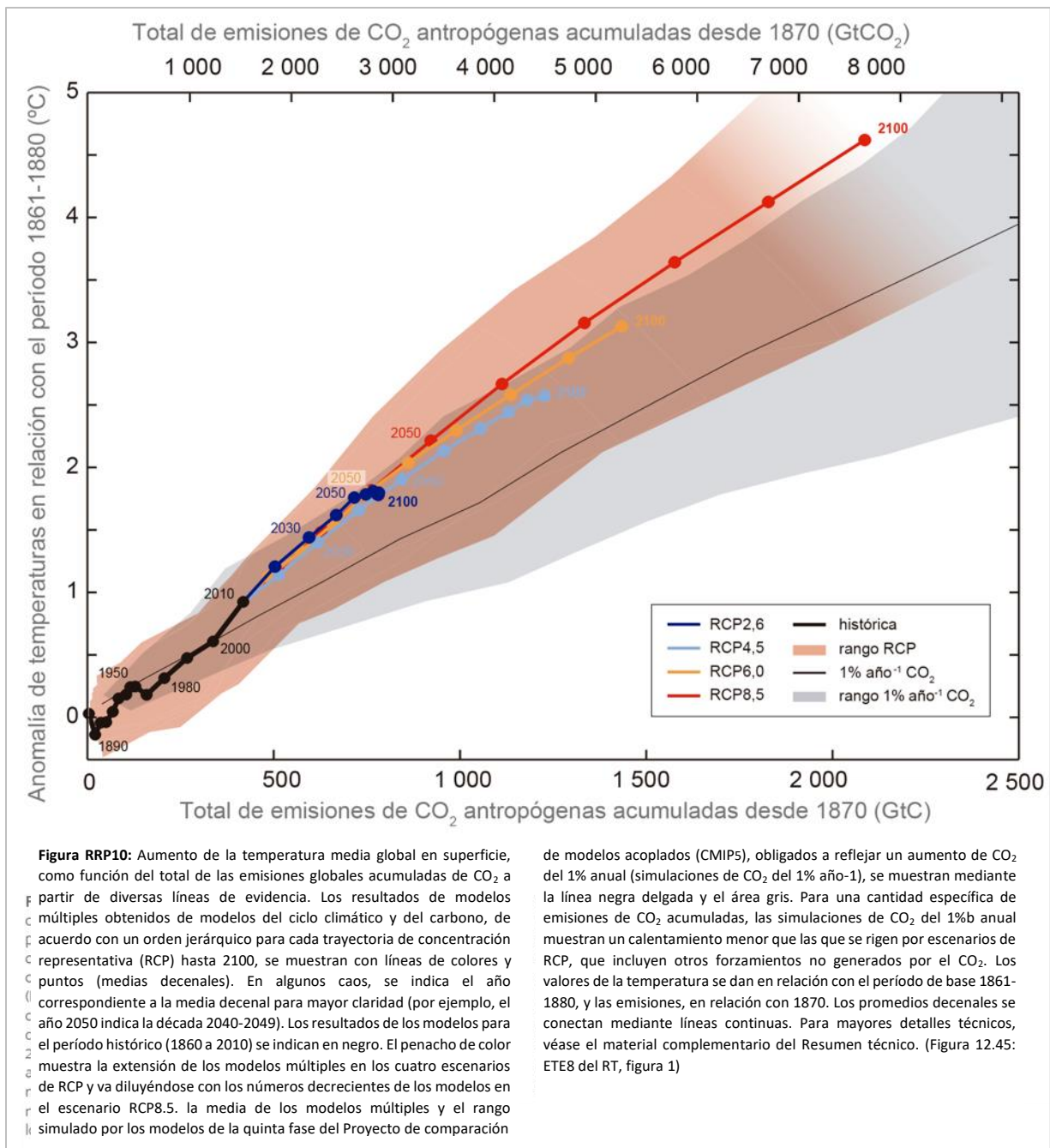
Figura 4. Emisiones antropógenas acumuladas Fuente. Climate Change Informe 3 IPCC 2014
