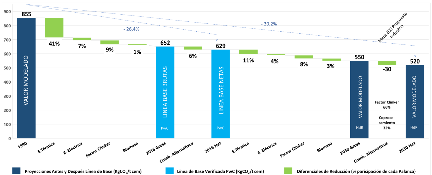
Figura 24. Participación de cada paper aplicado en la reducción de emisiones de CO 2 , proyectados antes y después al año base 2016. Alcance 1 Emisiones Netas y Brutas
