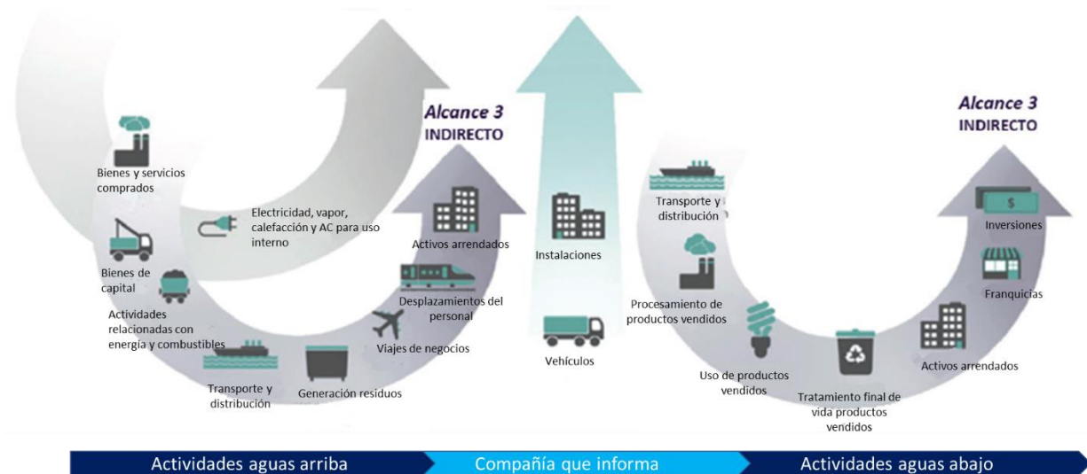
Figura 11. Alcances para la estimación de las emisiones Fuente. WBCSD
