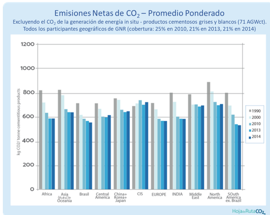
Figura 15. Ponderado de emisiones netas de CO 2 por región Fuente. GNR 2014
