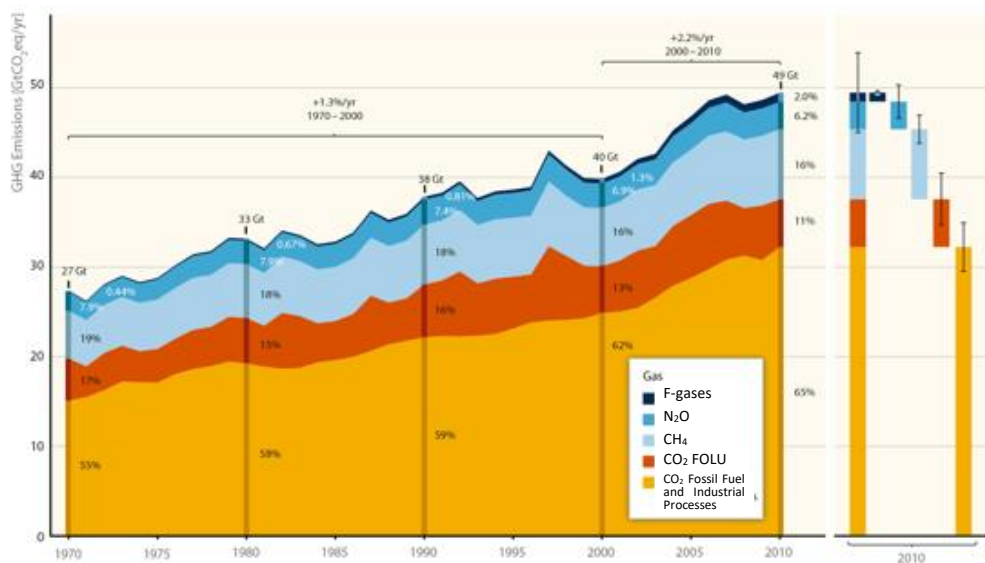
Figura RRP2: Emisiones antropógenas anuales totales de gases de efecto invernadero (GEI) (gigatonelada de CO 2 -equivalente al año, GtCO 2 -eq/año) para el período comprendido entre 1970 y 2010, por gases CO 2 procedente de la quema de combustibles fósiles y procesos industriales.; CO 2 procedente de la silvicultura y otros usos del suelo (FOLU); metano (CH 4 ); óxido nitroso (N 2 O); gases fluorados abarcados en el Protocolo de Kyoto. A la derecha se muestran las emisiones de 2010, con ponderaciones de emisiones de CO 2 -equivalente basadas en valores de los Informes de Evaluación segundo y quinto del IPCC. A menos que se indique de otro modo, las emisiones de CO 2 -equivalente en el presente
